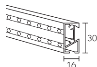
313100 Profil Perfil Profil
