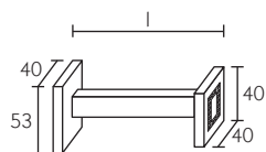
5130-- Fermatenda Holdback Porte-embrasse
