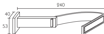
513064 Fermatenda bracciale Tieback Porte-embrasse-patère
